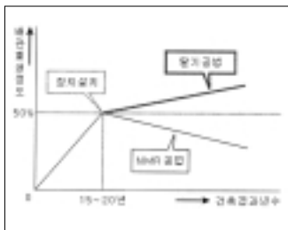
2. NMR
