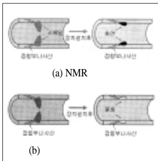
3. NMR
