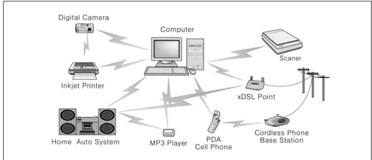
그림1. 블루투스 구성도
