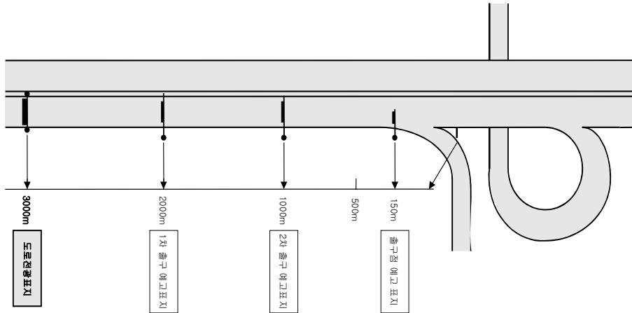
<그림 6.7> 지방부 고속도로 본선의 설치 지점 예시
