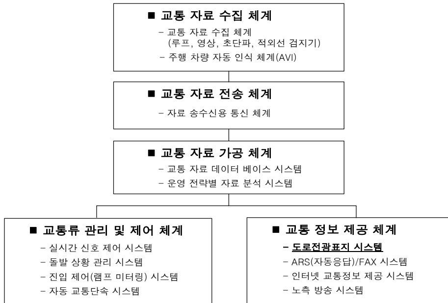
<그림 6.22> 첨단 교통관리체계 구성
