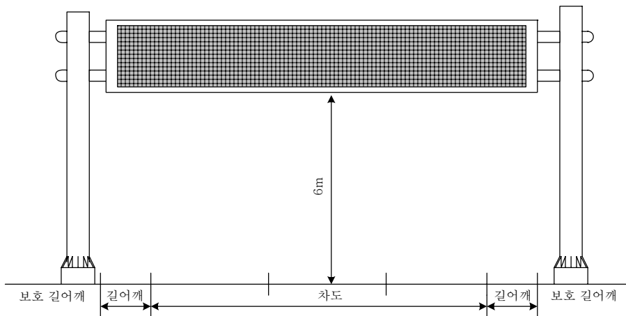
<그림 6.16> 문형식
