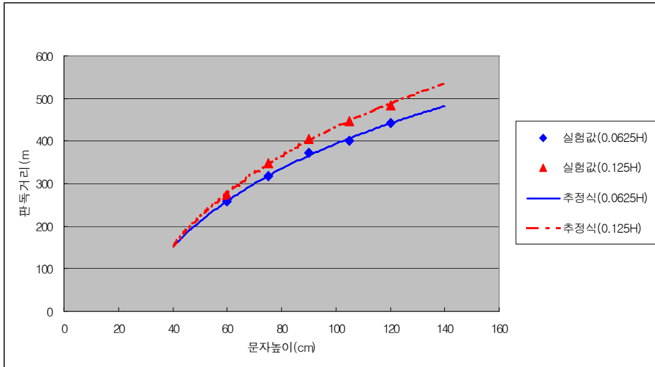
<그림 6.11> 문자 높이별 판독 가능 거리
