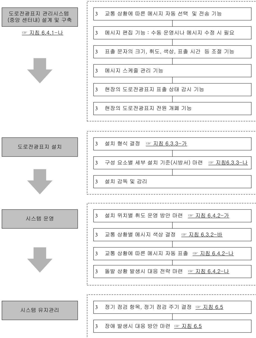
<그림 6.24> 도로전광표지 구축 과정(계속)
