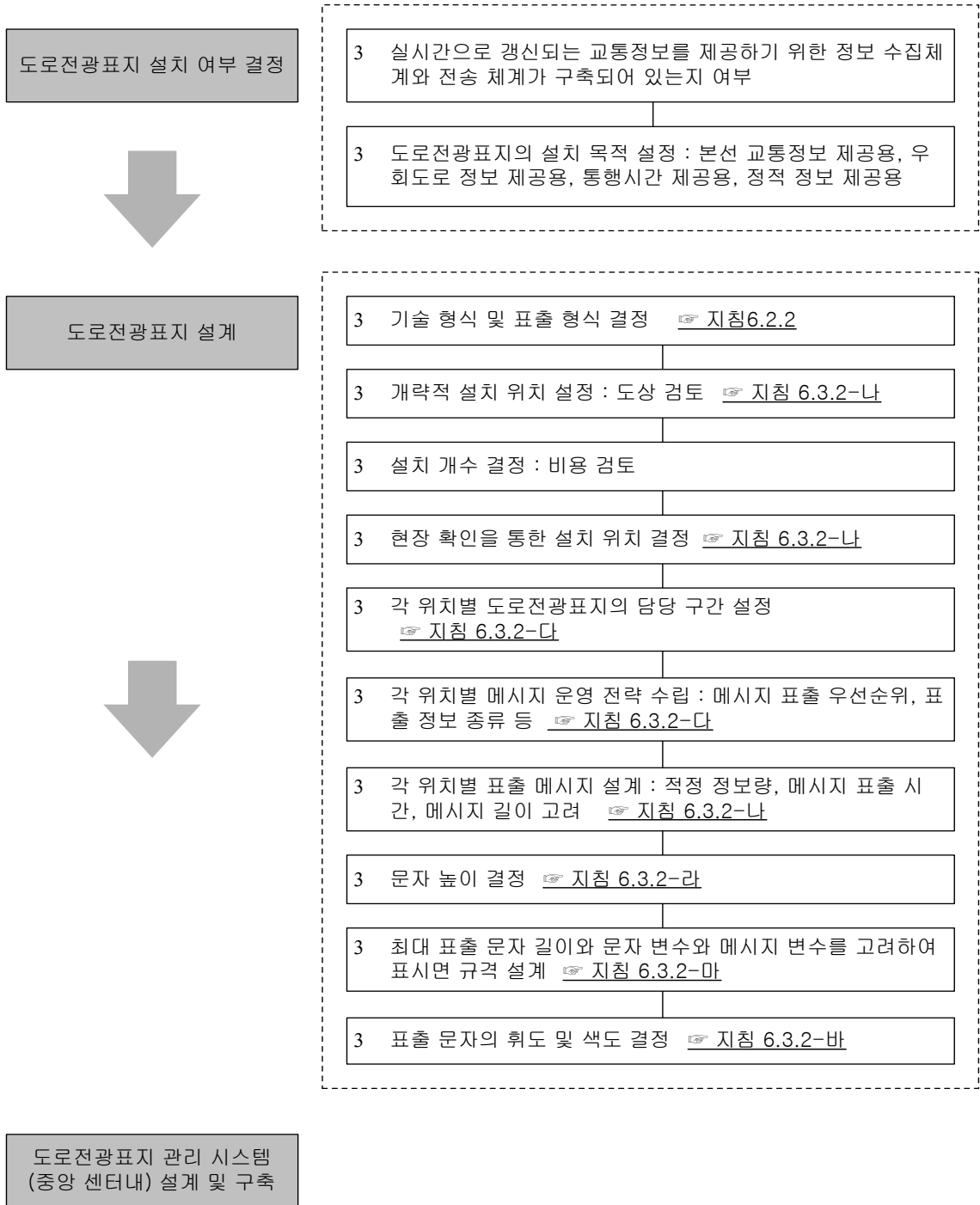
<그림 6.24> 도로전광표지 구축 과정
