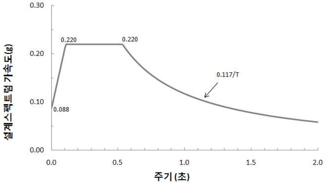
(a) 지진지역 1의 설계스펙트럼가속도
