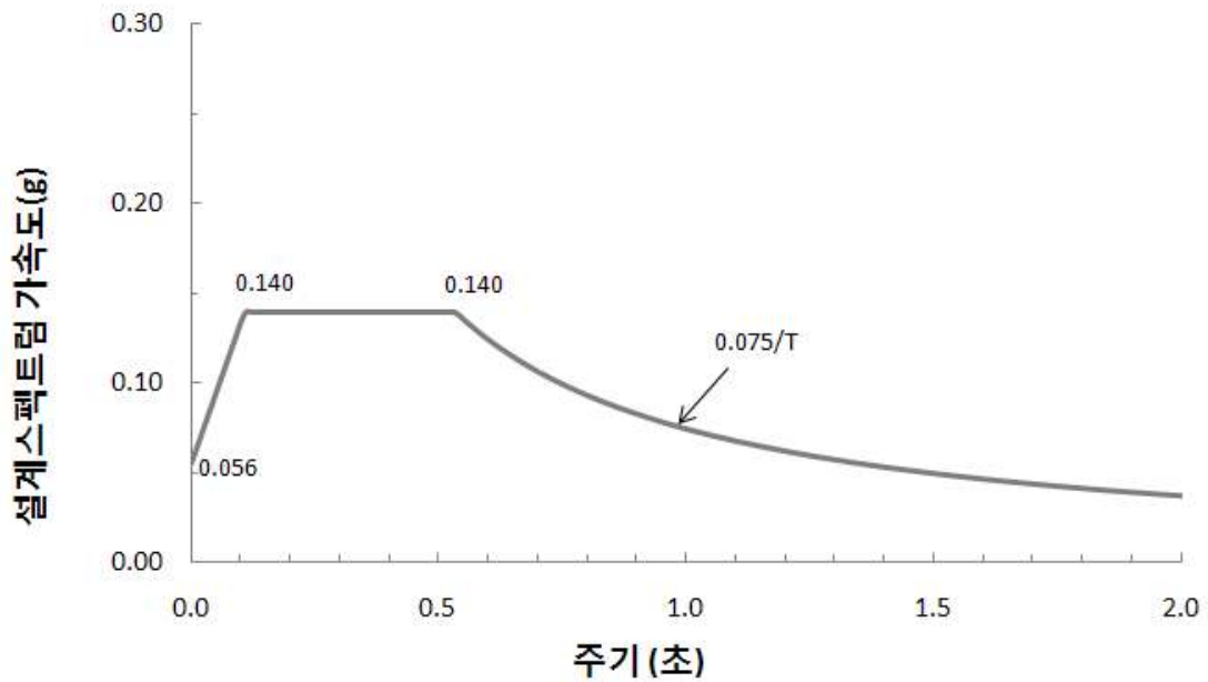
(b) 지진지역 2의 설계스펙트럼가속도
